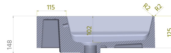
Sektion A-A
